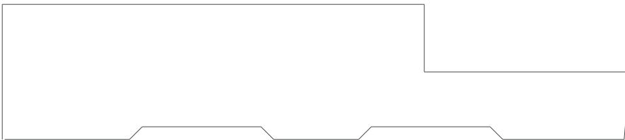
6700 Jamb 1.000" x 4.625"
