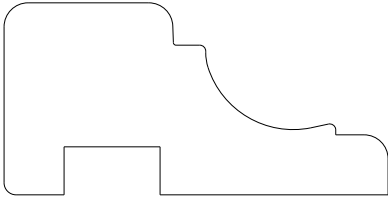
7584 Molding 1.000" x 2.000"
