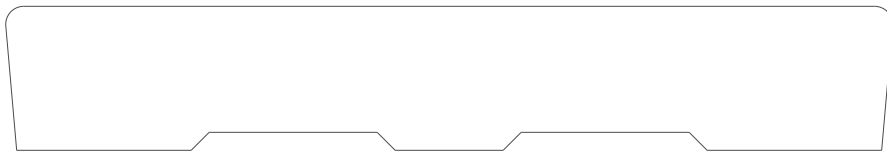
6400 Jamb 0.750" x 4.625"
