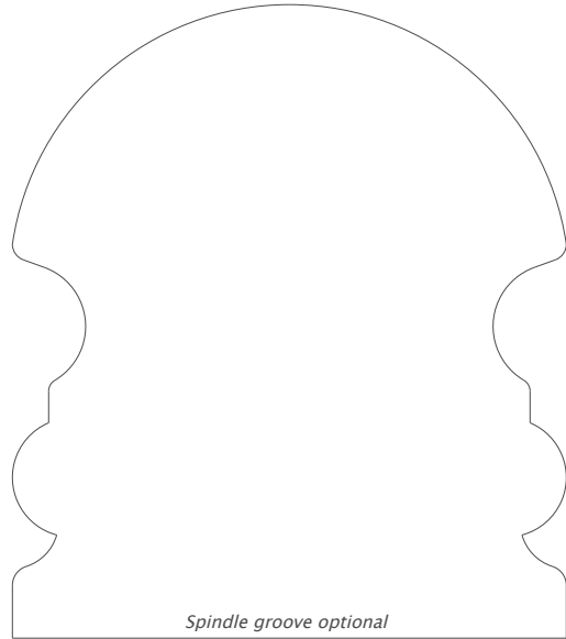
4550 Handrail 3.000" x 2.625"
