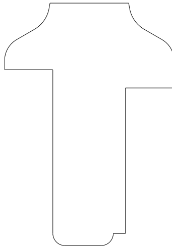
7011 Astragal 2.500" x 1.750"
