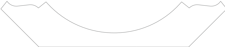
2567 Crown 1.000" x 5.000"
