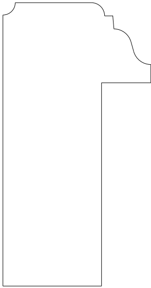
1506 Backband 1.500" x 2.875"
