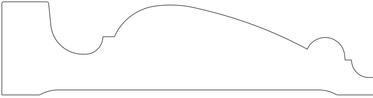
1554 Casing 1.000" x 4.000"
