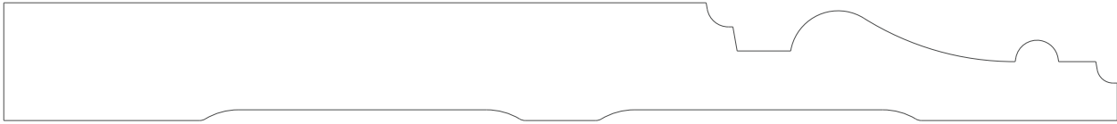
3036 Base 0.687" x 6.500"
