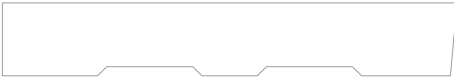
6110 Jamb 0.750" x 4.625"
