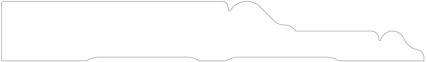
3038 Base 1.000" x 7.000"
