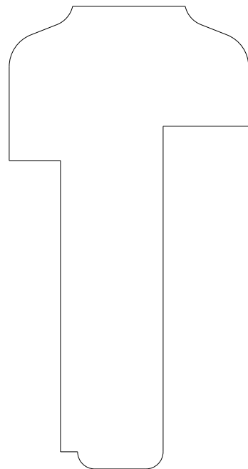
7042 Astragal 3.375" x 1.750"
