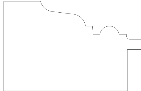
1581 Backband 1.625" x 2.500"
