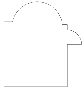
1512 Backband 1.500" x 1.375"
