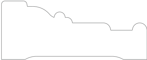
1530 Casing 1.000" x 2.500"
