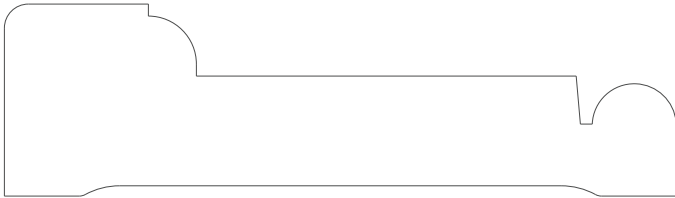
1207 Casing 1.000" x 3.500"
