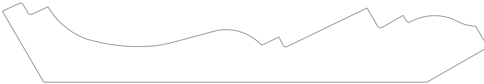
2059 Crown 0.812" x 5.000"
