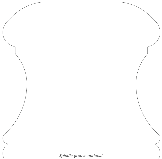
4563 Handrail 3.500" x 3.500"
