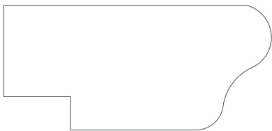
6074 Sill 0.937" x 2.000"
