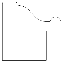
1091 Backband 1.000" x 1.000"
