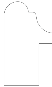
1510 Backband 1.500" x 0.875"
